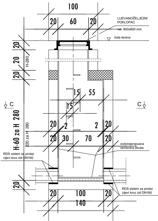
PRESJEK A-A
