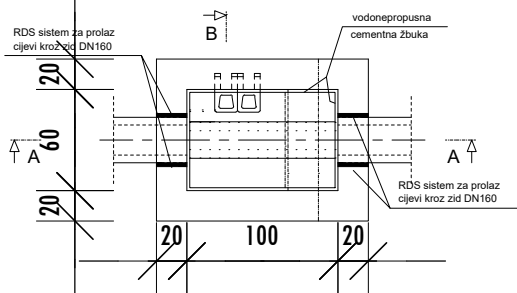
TLOCRT (C-C)
