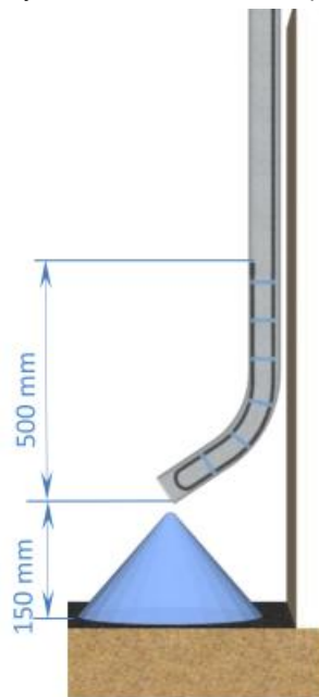
Slika 4: Grijanje vertikalnih odvođa (slika preuzeta iz kataloga ELPOS d.o.o.)
