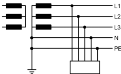
Slika: TN-S sustav mreže
