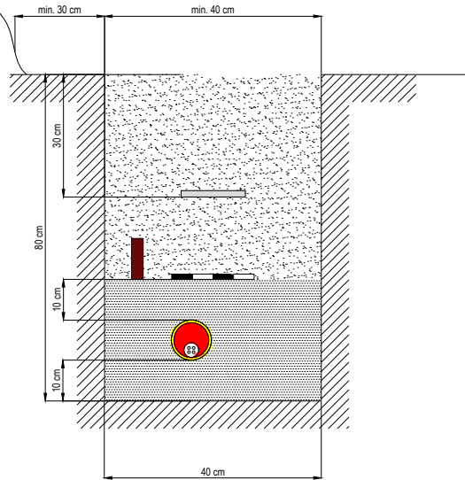
Presjek kabelskog rova za polaganje kabela nazivnog napona U_0/U = 1 kV
