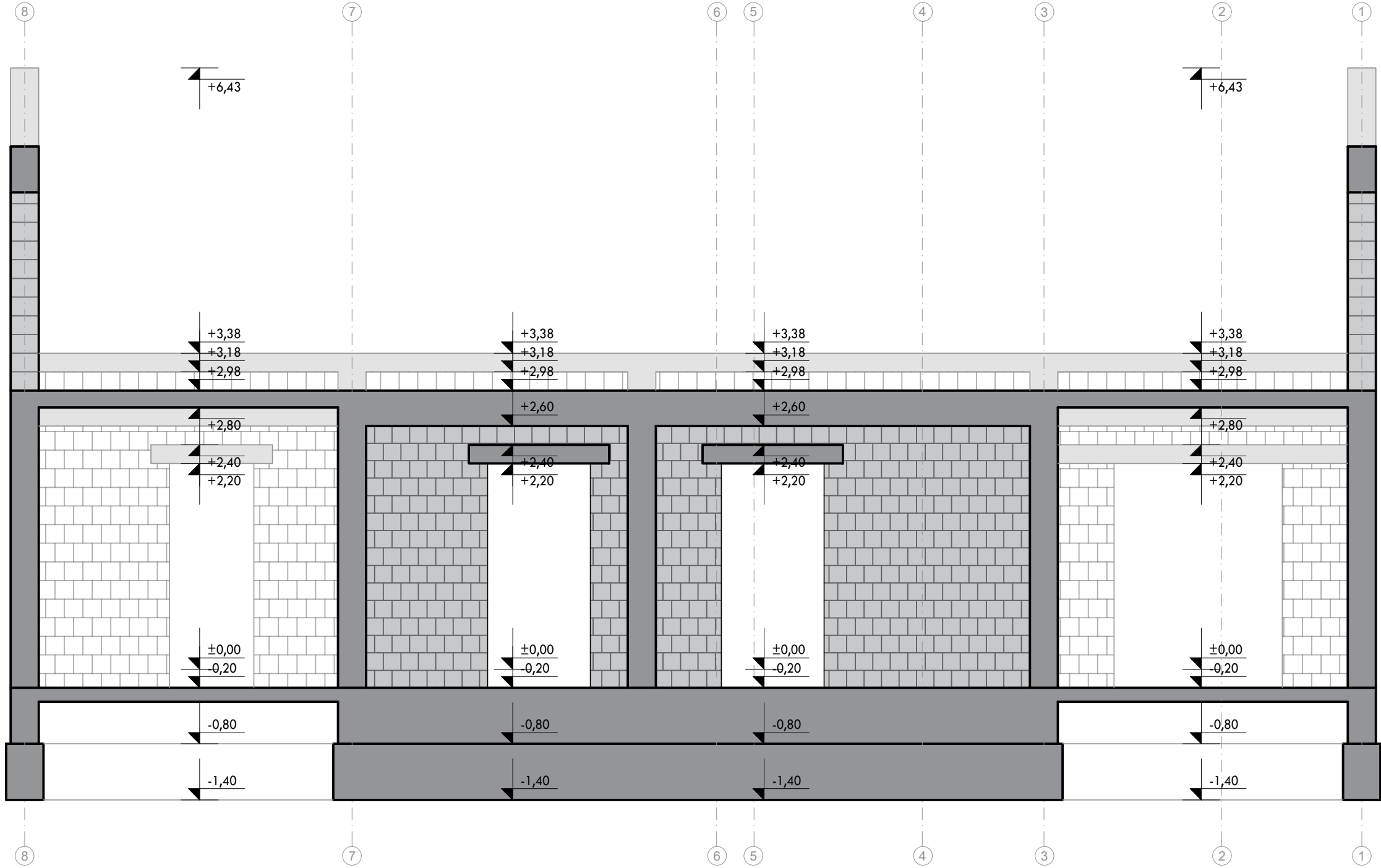
OS B-B
