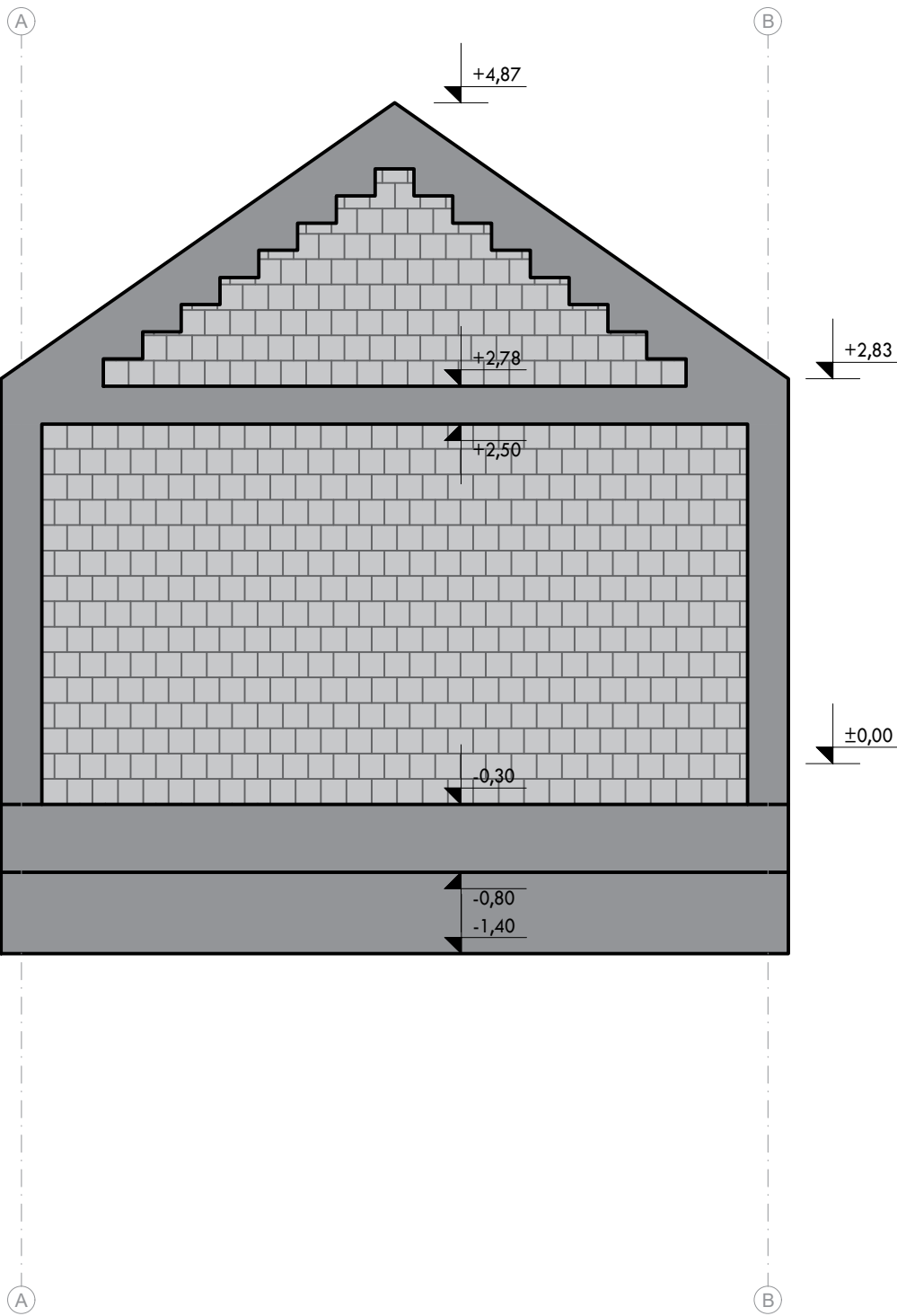
OS 4-4
