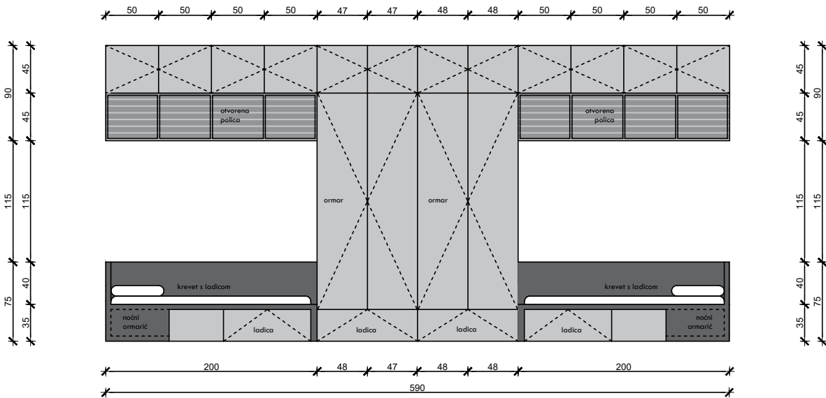
POGLED
