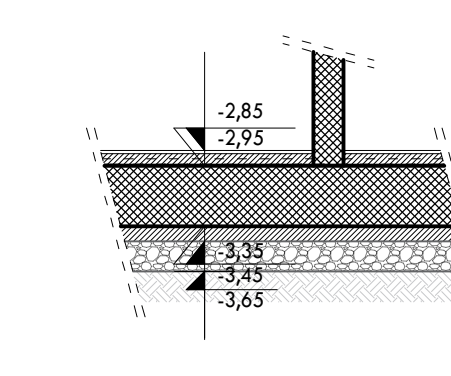
PRESJEK 17_17
