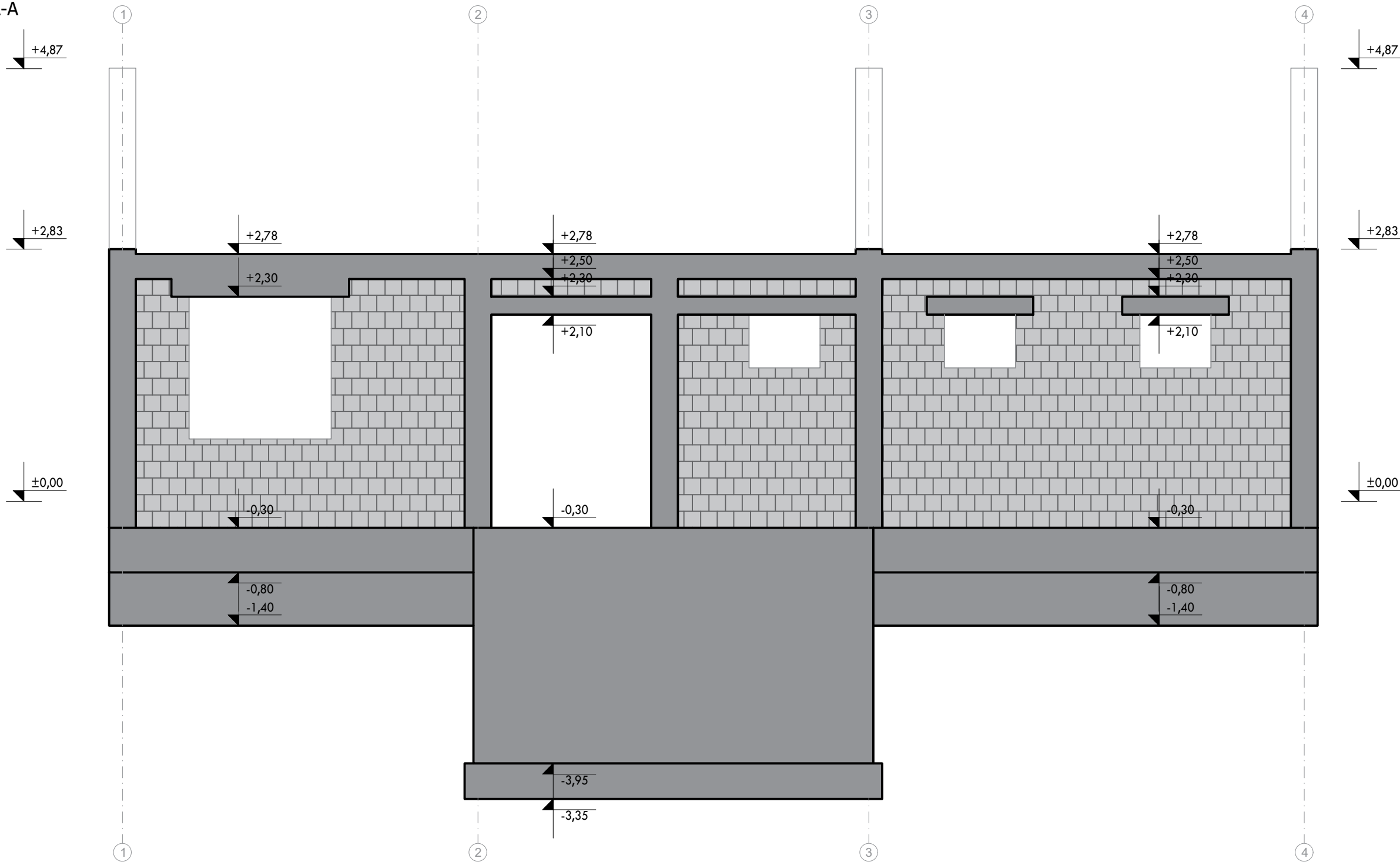
OS B-B
