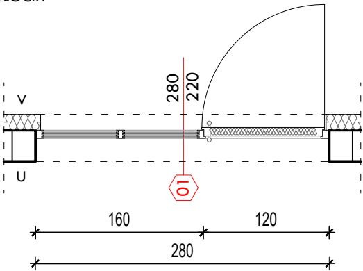
TLOCRT
