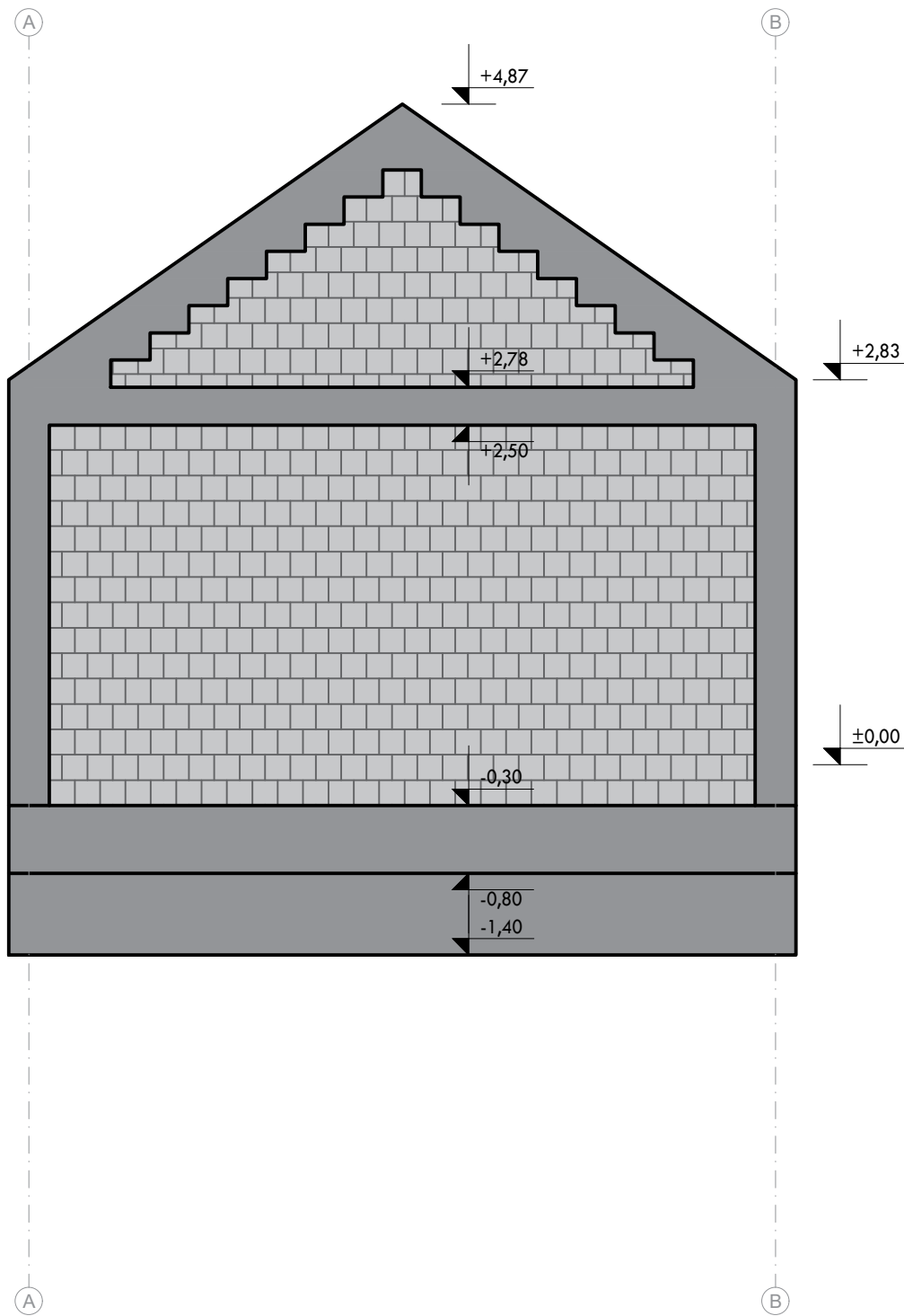
OS 1-1
