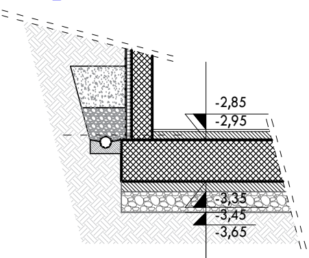
PRESJEK 16_16
