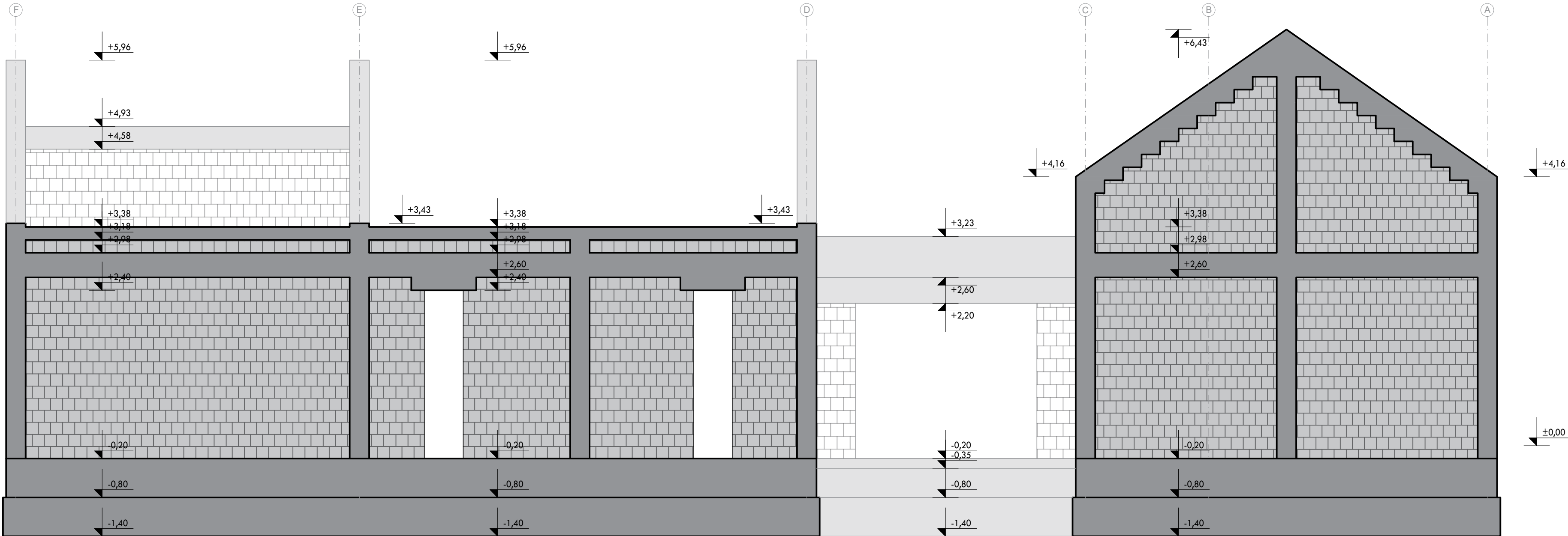
OS 1-1
