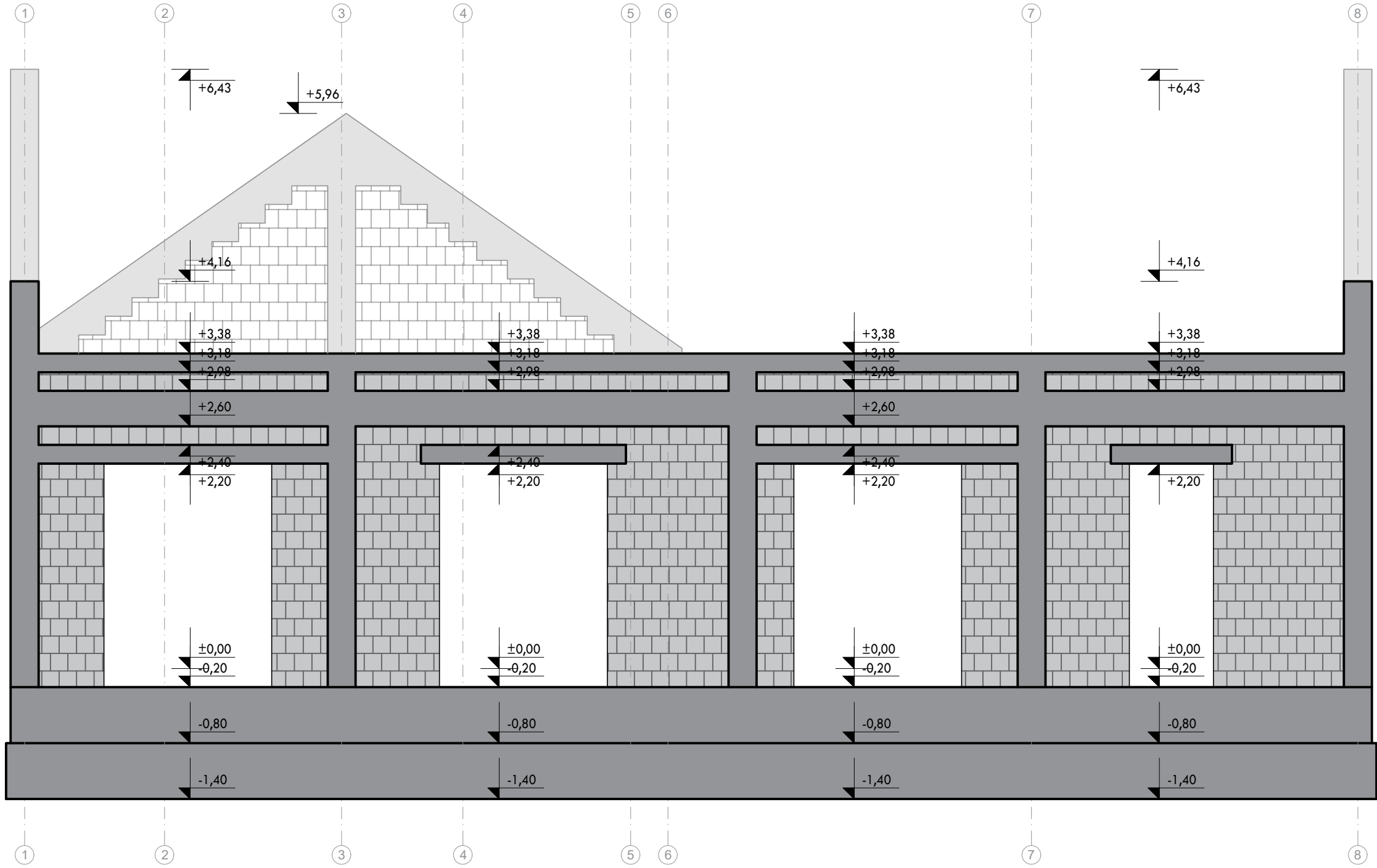
OS A-A
