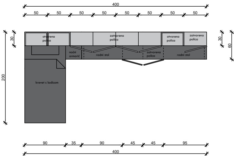
TLOCRT
