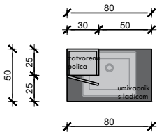
TLOCRT
