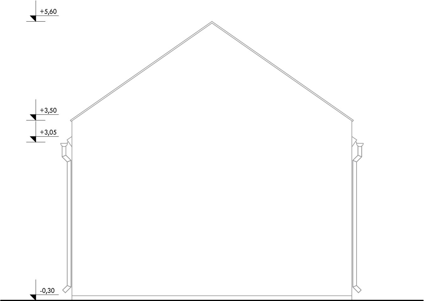
JUGOZAPADNO PROČELJE
