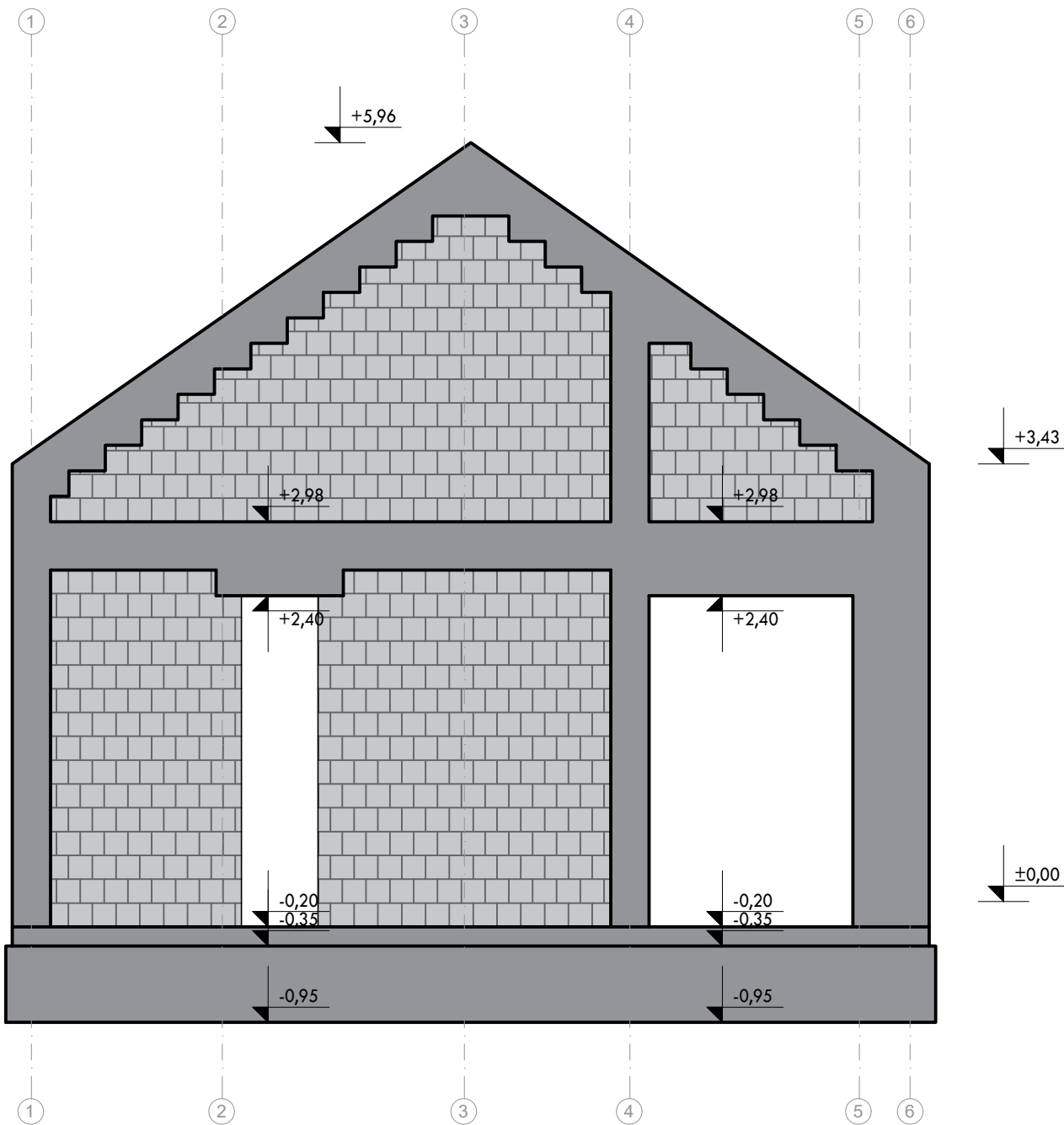
OS F-F
