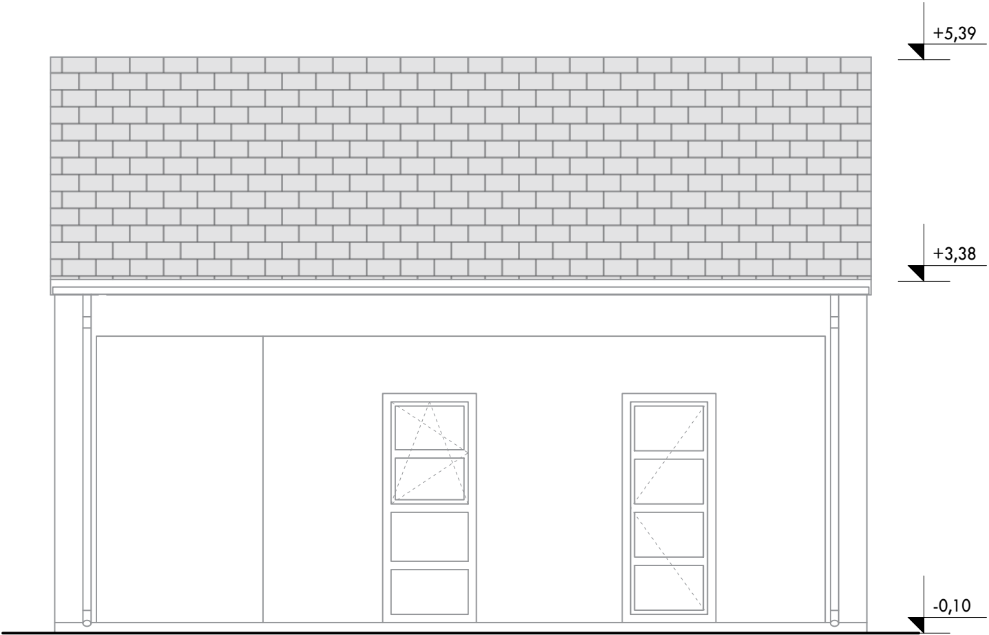
zapadno pročelje
