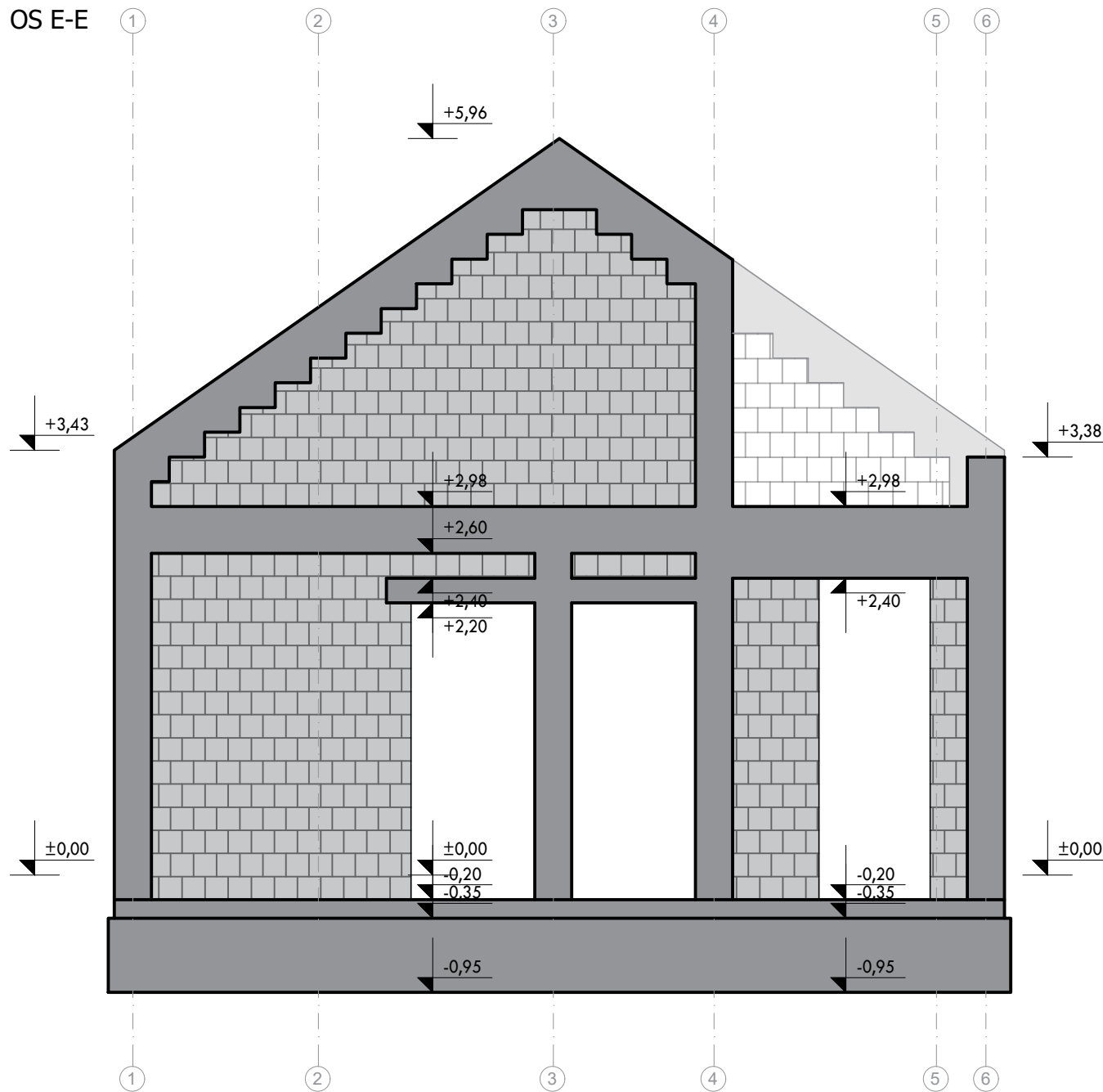
OS E-E
