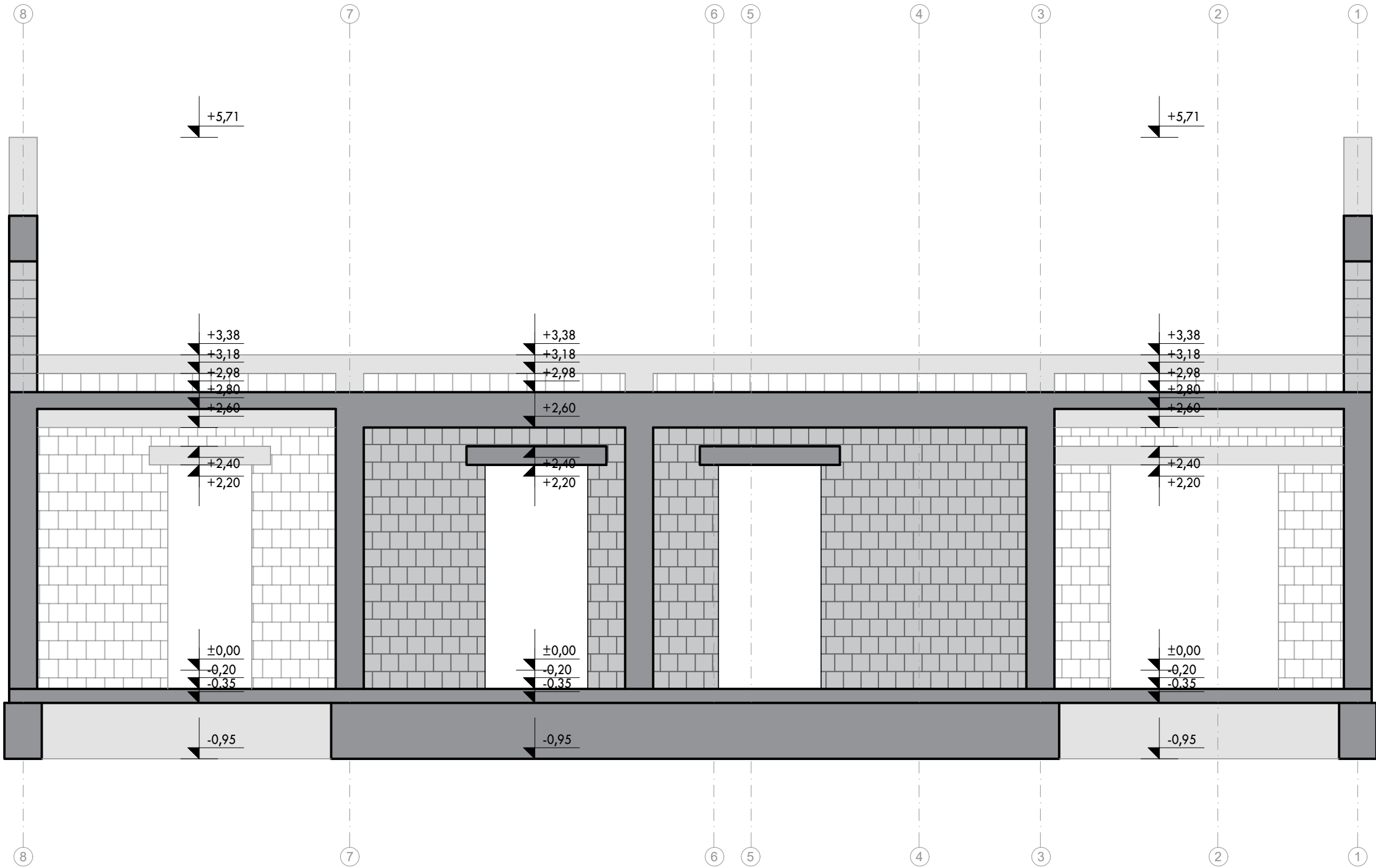
OS B-B
