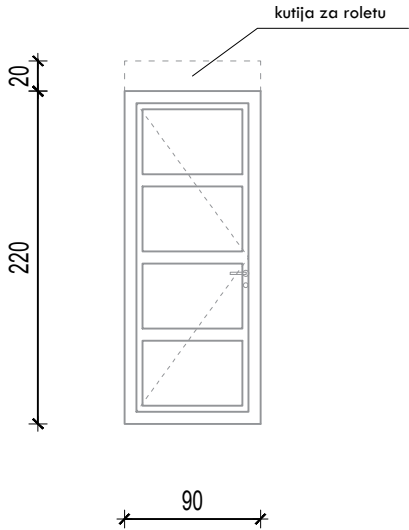
POGLED
