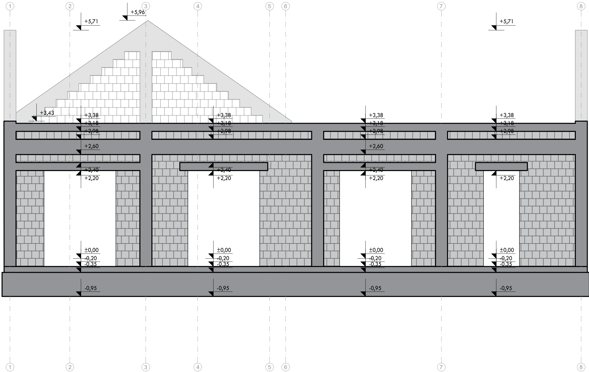
OS A-A
