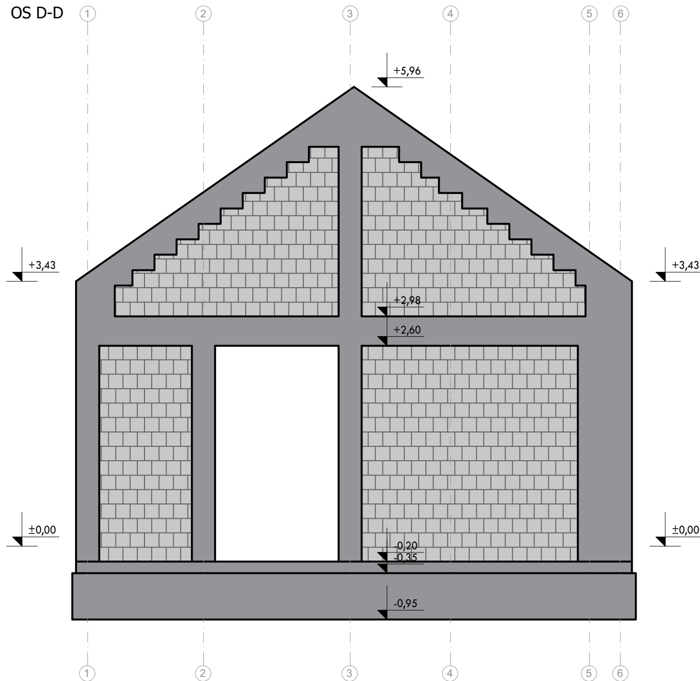
OS D-D
