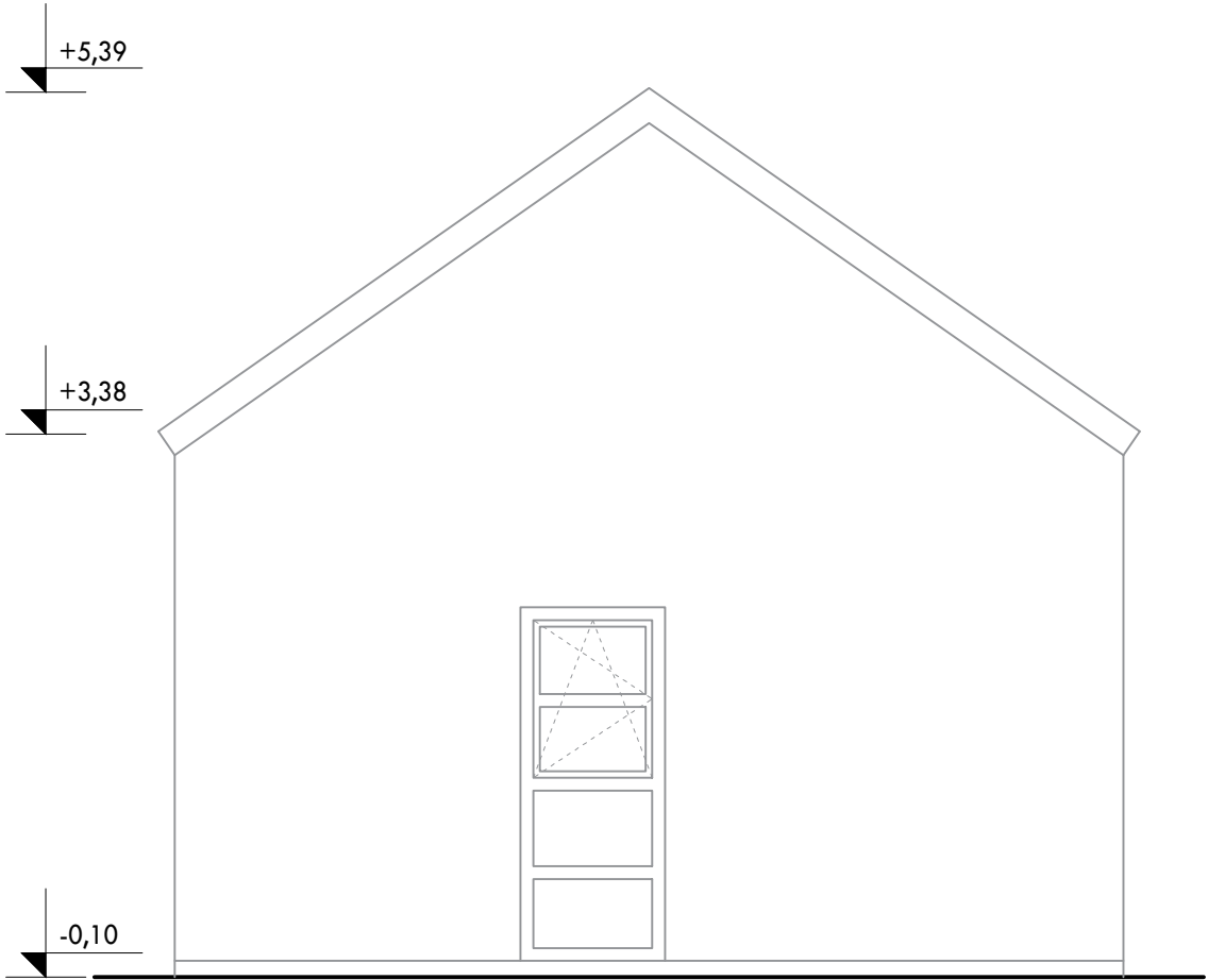
južno pročelje
